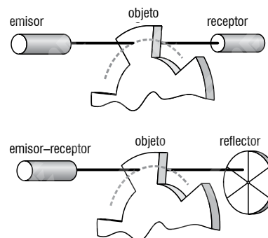
Fig. 18: Los modos en barrera y reflex: el haz de luz debe cortarse por el objeto
