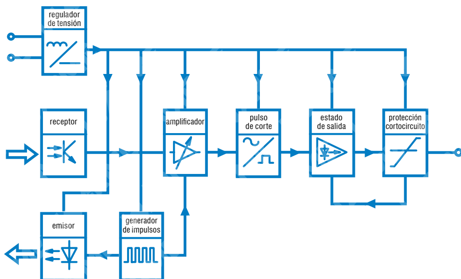
Fig. 8: Bloques funcionales de un sensor fotoeléctrico
